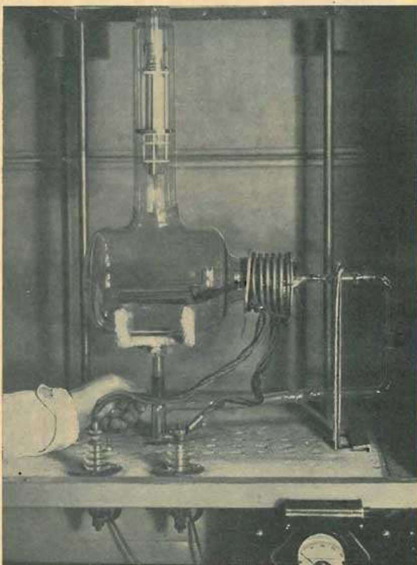
Telopantoscopia Safar (Tubo a raggi catodici trasmettente per telecinema) sul banco di vuotatura. Costruito con brevetti italiani.
